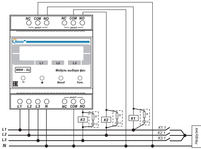
Рис.2. Схема подключения МВФ-3Ц для работы с мощной нагрузкой. Необходимо включать параллельно катушке пускателя искрогасящую цепочку R – 51 Ом 1Вт, С – 0,1 мкФ 630 В.
